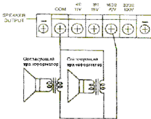
Подключение нагрузки 16Ω
